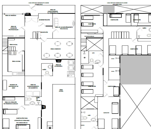
Imagen No.2. Planos correspondientes a la casa refugio MANUELITA SÁENZ ubicada en la localidad Teusaquillo barrio la Soledad, Cra. 27a No.42-36 bajo la ejecución del contrato 566 de 2020
